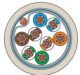
F/UTP
